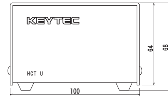
正面図
